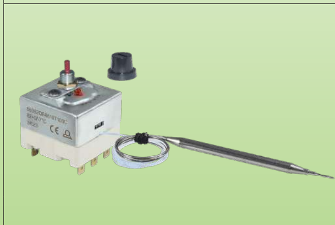
1. sellado; 2. Manga; 3. Botón de restablecimiento manual; 4. Tapa de plástico (Negro)
