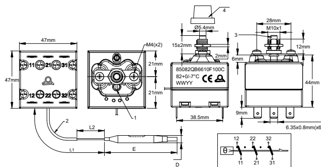
1. sellado; 2. Manga; 3. Botón de restablecimiento manual; 4. Tapa de plástico (Negro)
