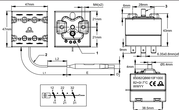
1. sellado; 2. Manga; 3. Botón de restablecimiento manual
